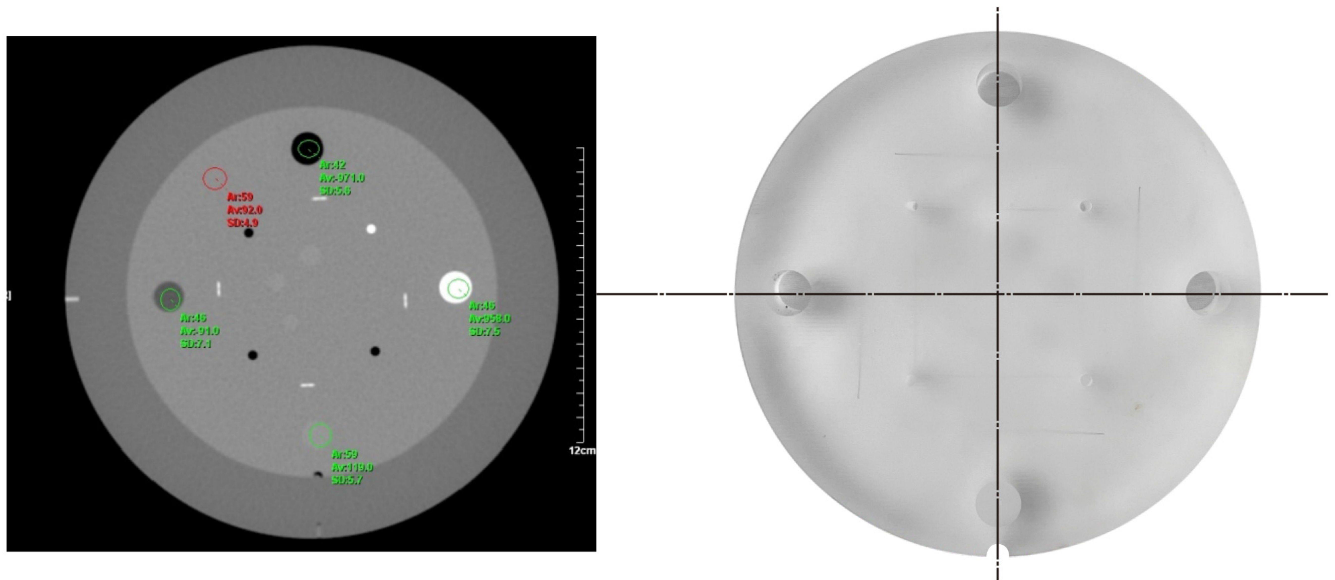
图 A.1 测试 Z 轴对准的精度
